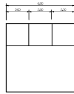
Visão frontal
